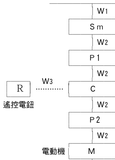
圖 153：標準電動機分路圖
